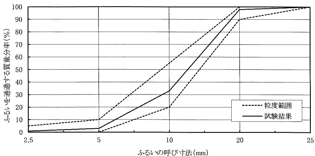
粒度分布曲線
